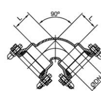
Coude Double Emboîtement 90°
